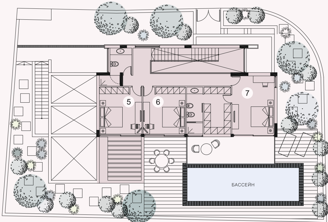
ВТОРОЙ ЭТАЖ
