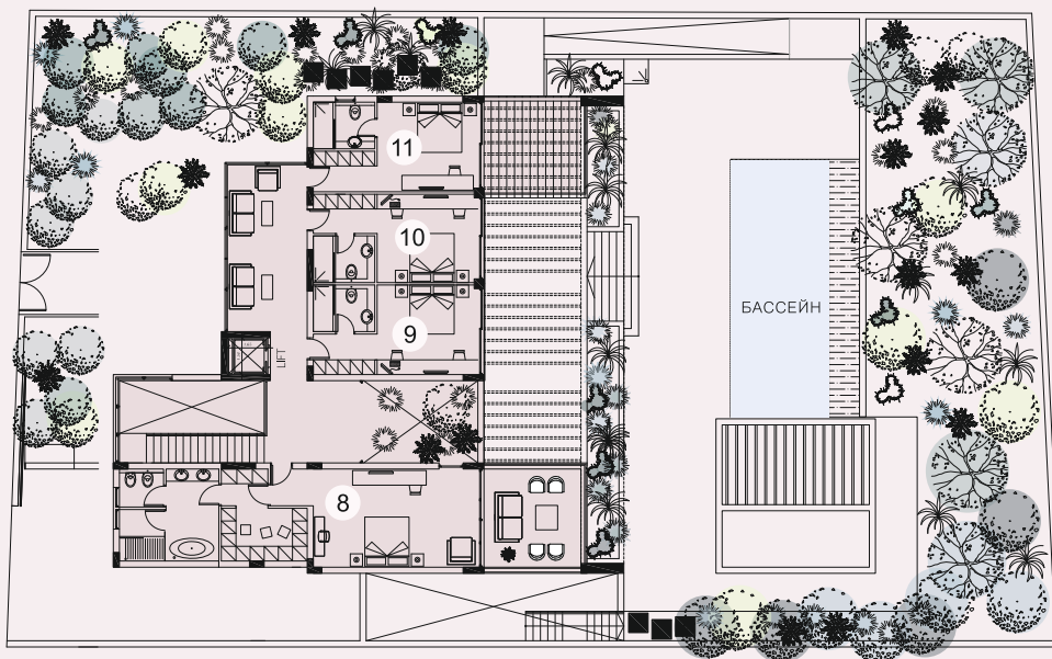
ВТОРОЙ ЭТАЖ
