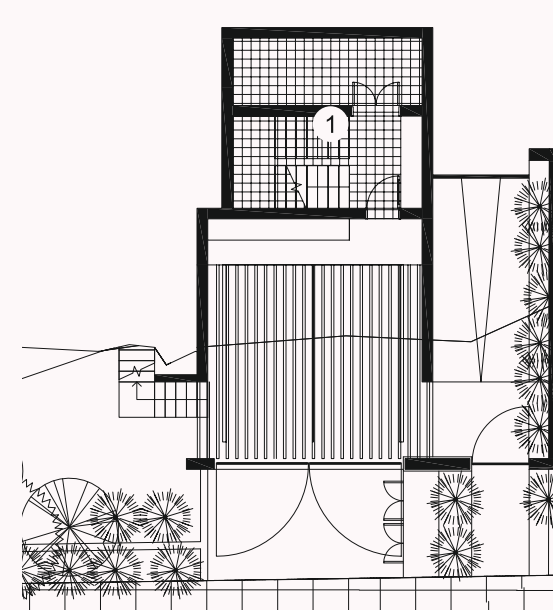
ЦОКОЛЬНЫЙ ЭТАЖ
