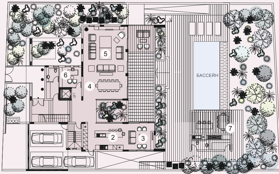
ПЕРВЫЙ ЭТАЖ
