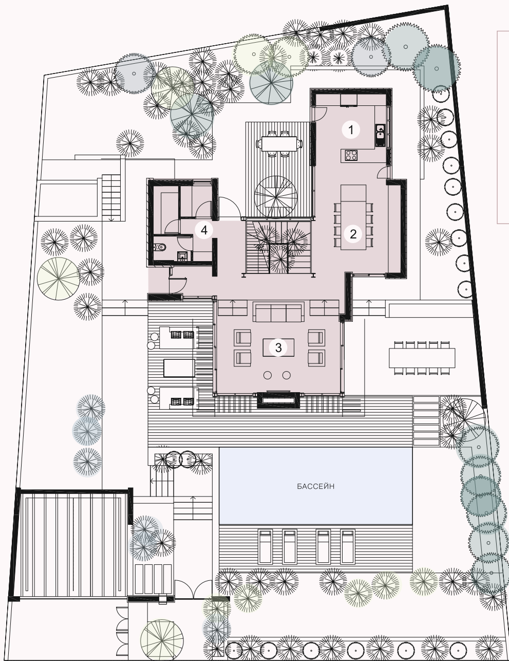
ПЕРВЫЙ ЭТАЖ
