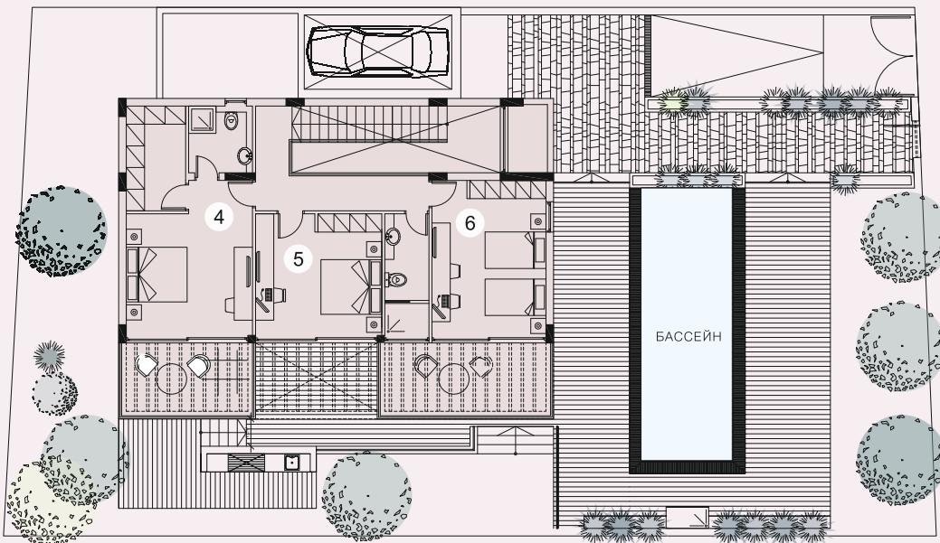
ВТОРОЙ ЭТАЖ
