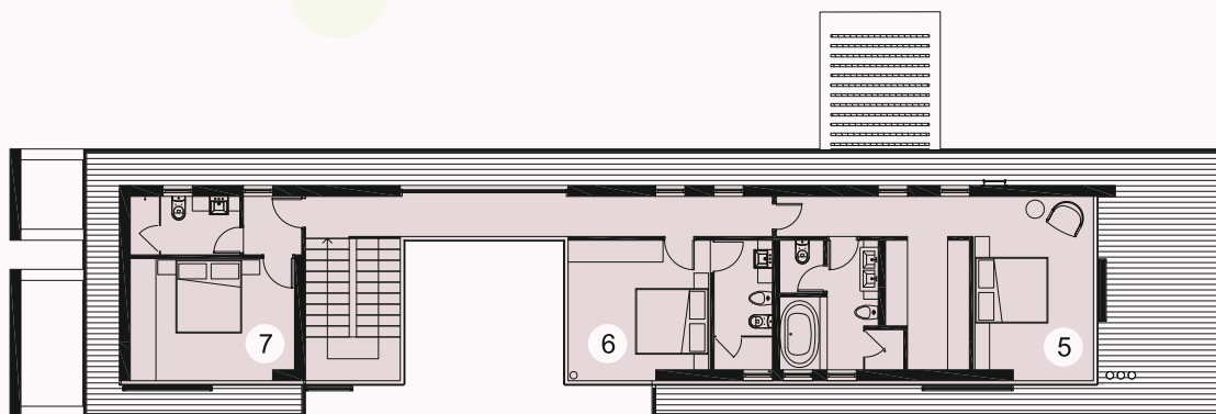
ПЕРВЫЙ ЭТАЖ
