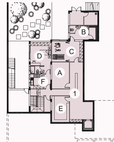
ЦОКОЛЬНЫЙ ЭТАЖ
