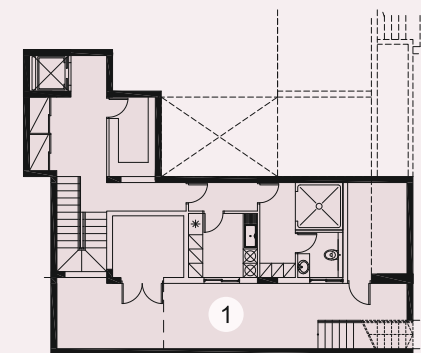
ЦОКОЛЬНЫЙ ЭТАЖ
