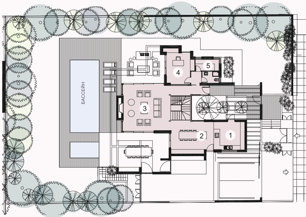
ПЕРВЫЙ ЭТАЖ
